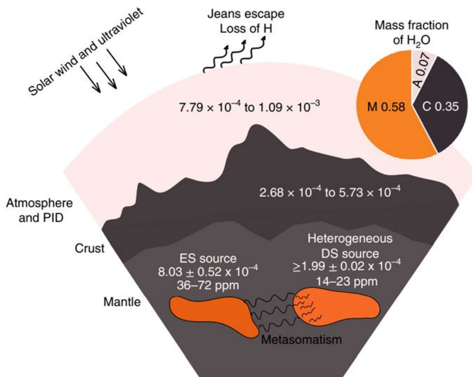
Рис. 6. Схематическое изображение двух изотопных резервуаров в марсианской мантии (рыжие пятна) и значения D/H в коре и атмосфере. В верхнем правом углу показано распределение H 2 O в различных геологических оболочках Марса (M — мантия, C — кора, A — атмосфера). Рисунок из обсуждаемой статьи в Nature Geoscience
